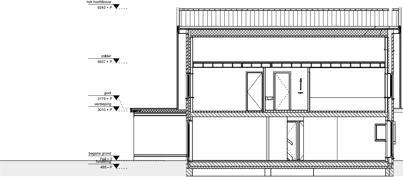
Doorsnede B-B
